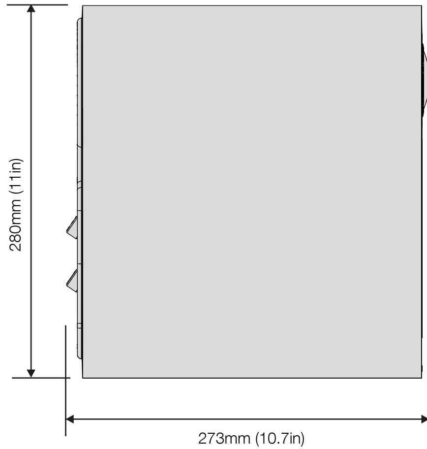
LEFT SIDE
