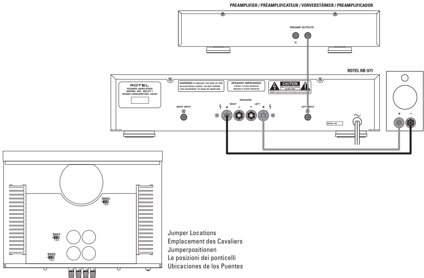
Figure 3: Bridged Mono Connections – Inputs and Speakers Branchements des entrées et des enceintes en ponté mode mono Anschlußdiagramm bei Brückenschaltung - Eingänge und Lautsprecher Collegamenti mono configurazione "a ponte" - Ingressi e diffusori Conexiones para el Funcionamiento en Modo Monofónico Puenteado - Terminales de Entrada y de Conexión a las Cajas Acústicas
