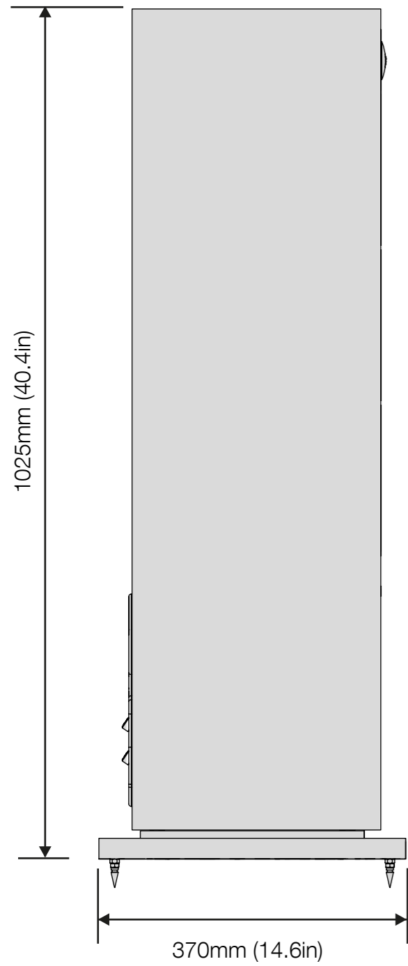
LEFT SIDE
